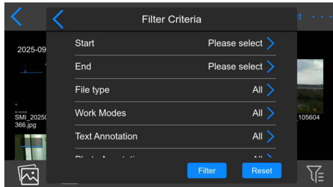
6.1.1.4-1-Criteria
