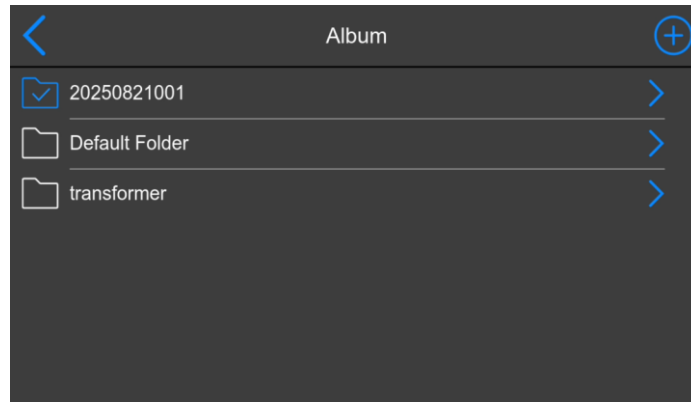
6.1.1-Album Interface
