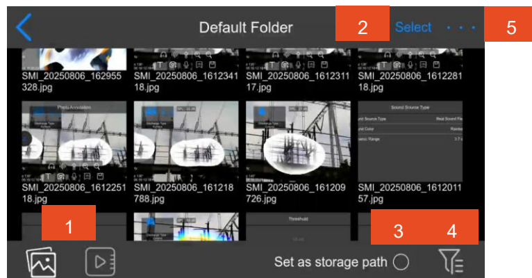
6.1.1.1-Folder Interface
